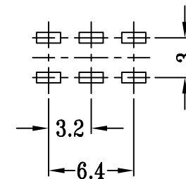
P.C.B LAYOUT
